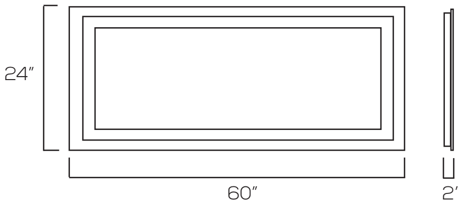
SES-ML01-6024-20W-S (80W)
